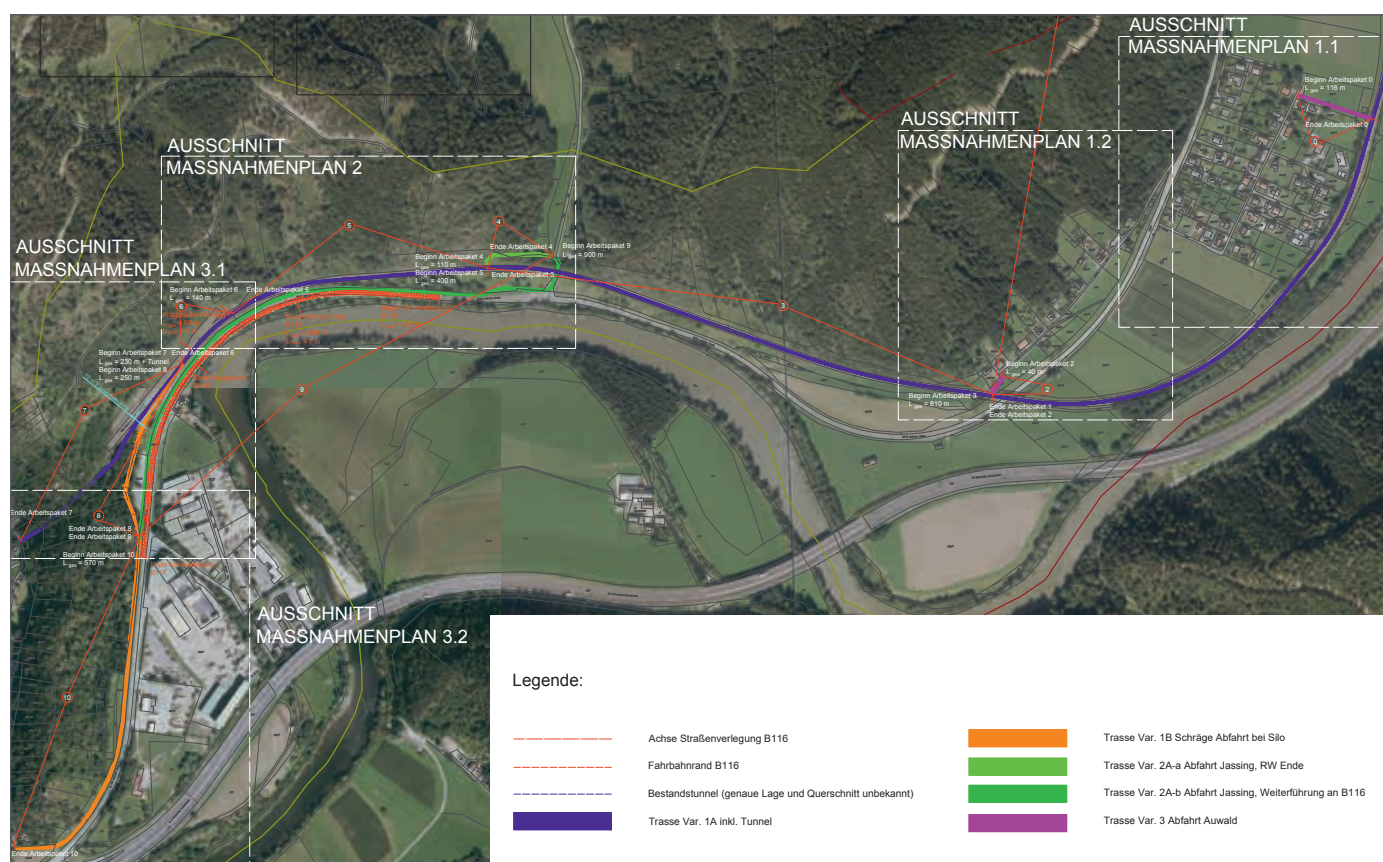
Überblick über die möglichen Trassen für die Fortsetzung des Radweges von der Stadtgrenze Leoben-Hinterberg nach St. Michael
